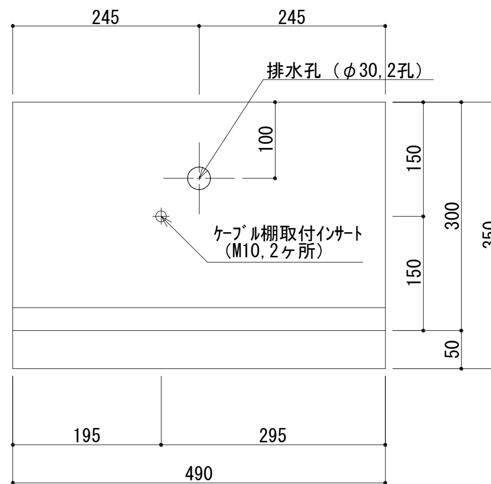
A-A 断面図
