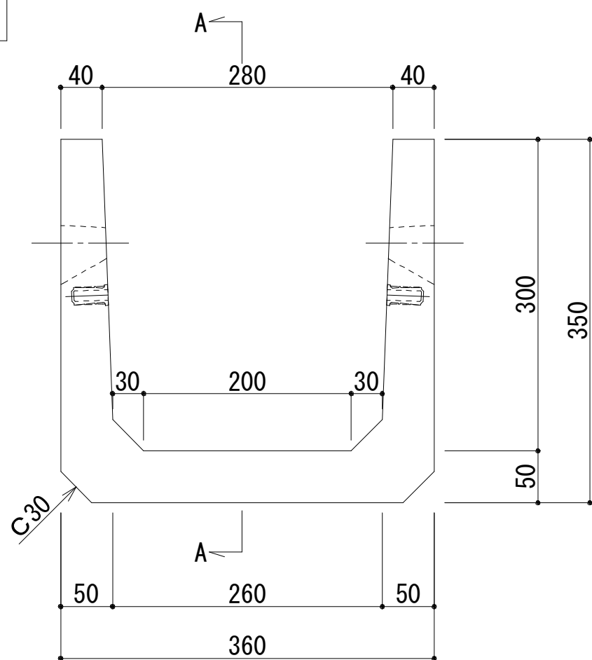
製品図
