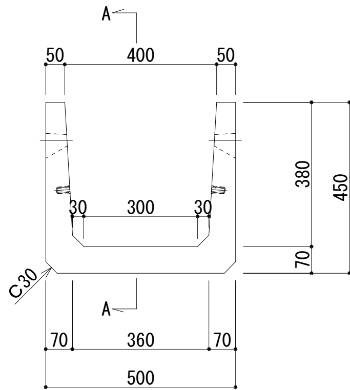
製品図
