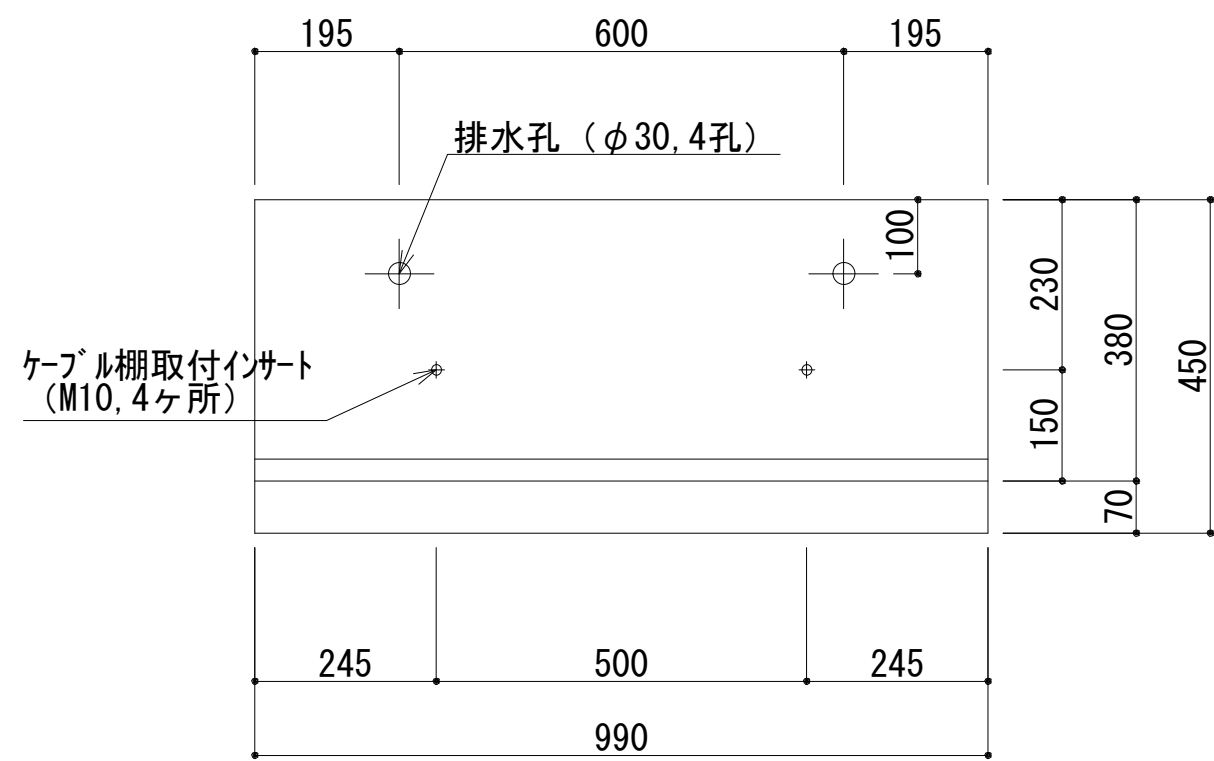
A-A 断面図
