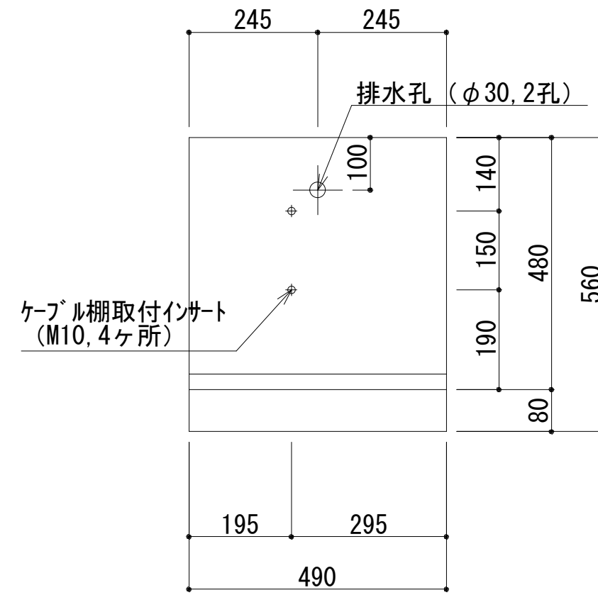
A-A 断面図
