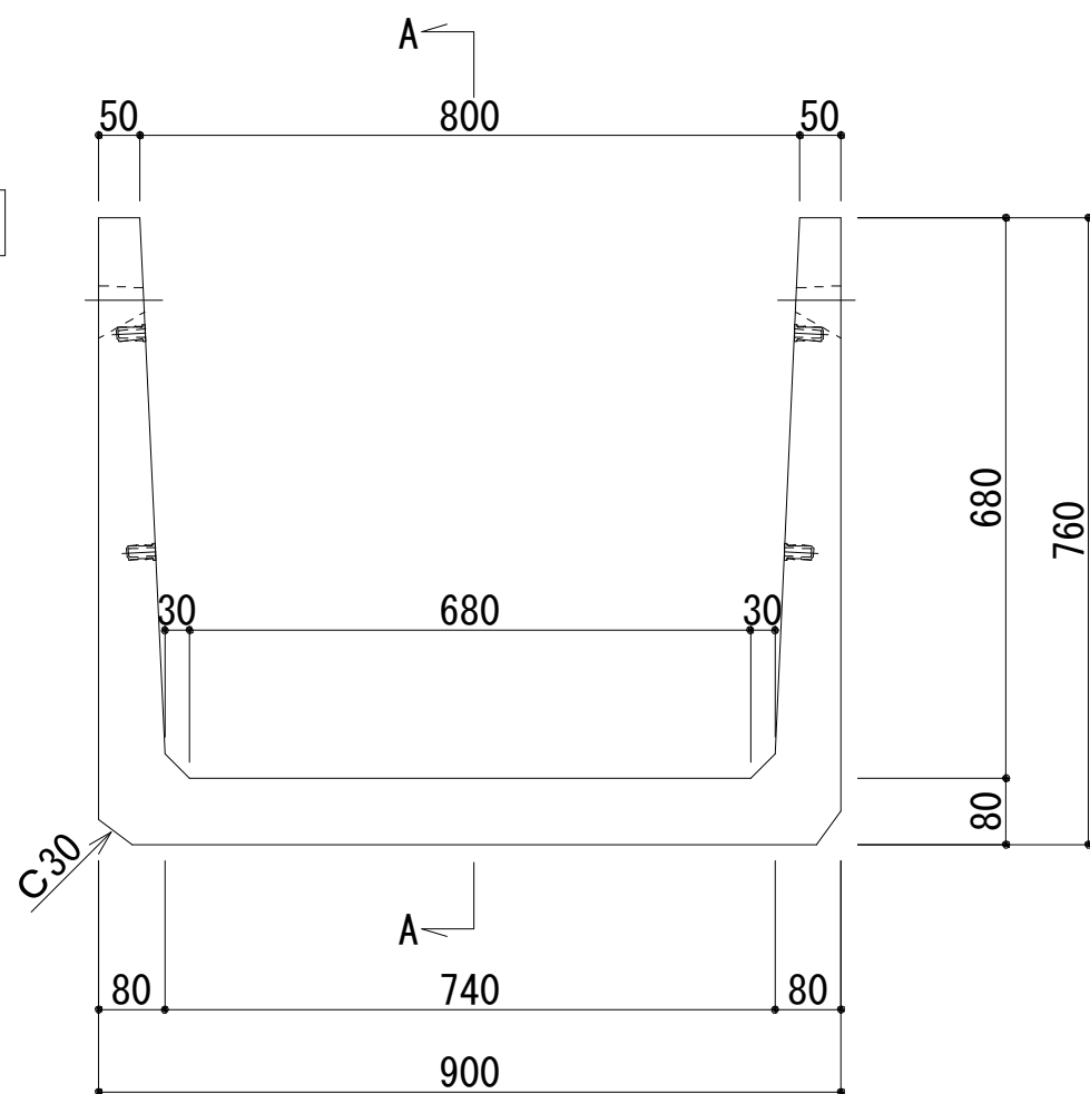
製品図
