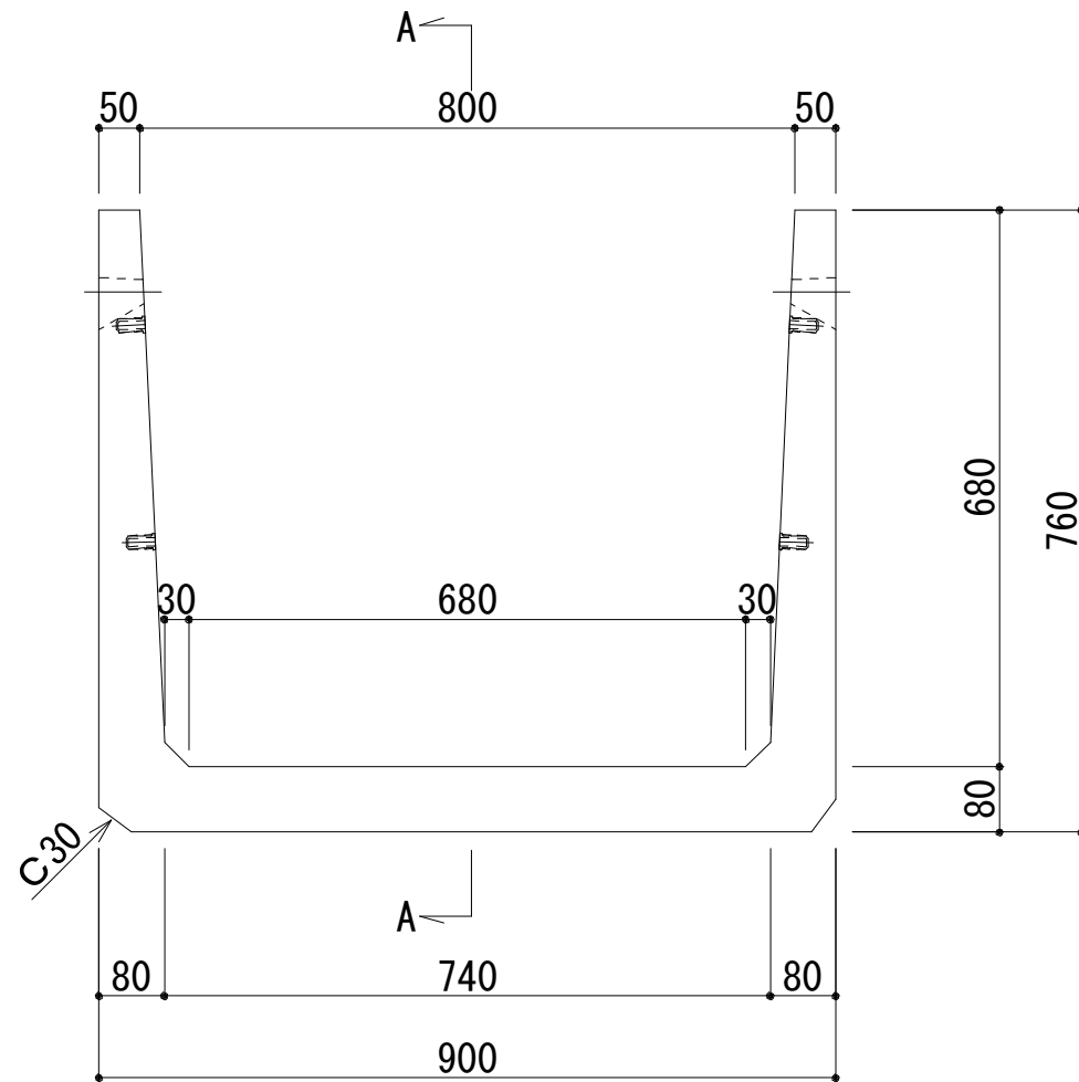
製品図
