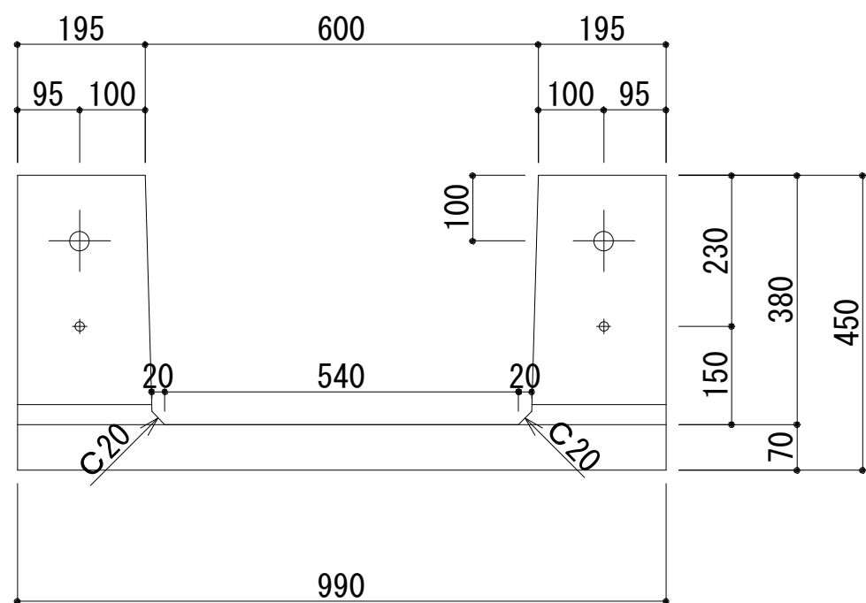
A-A 断面図
