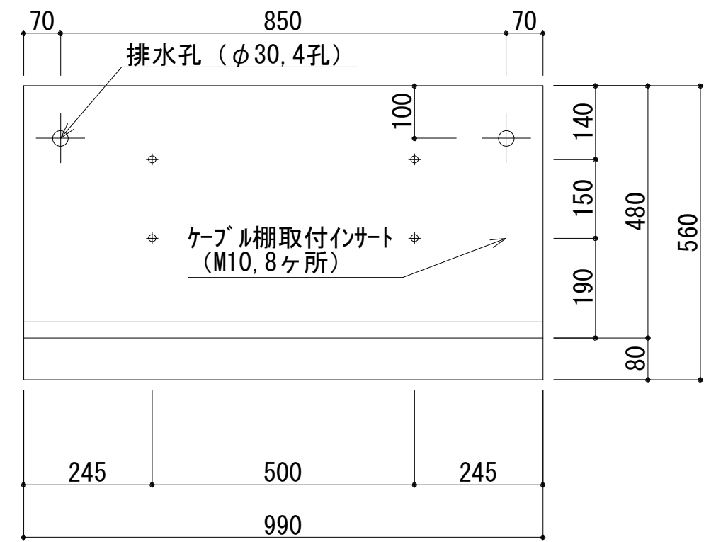
B-B 断面図
