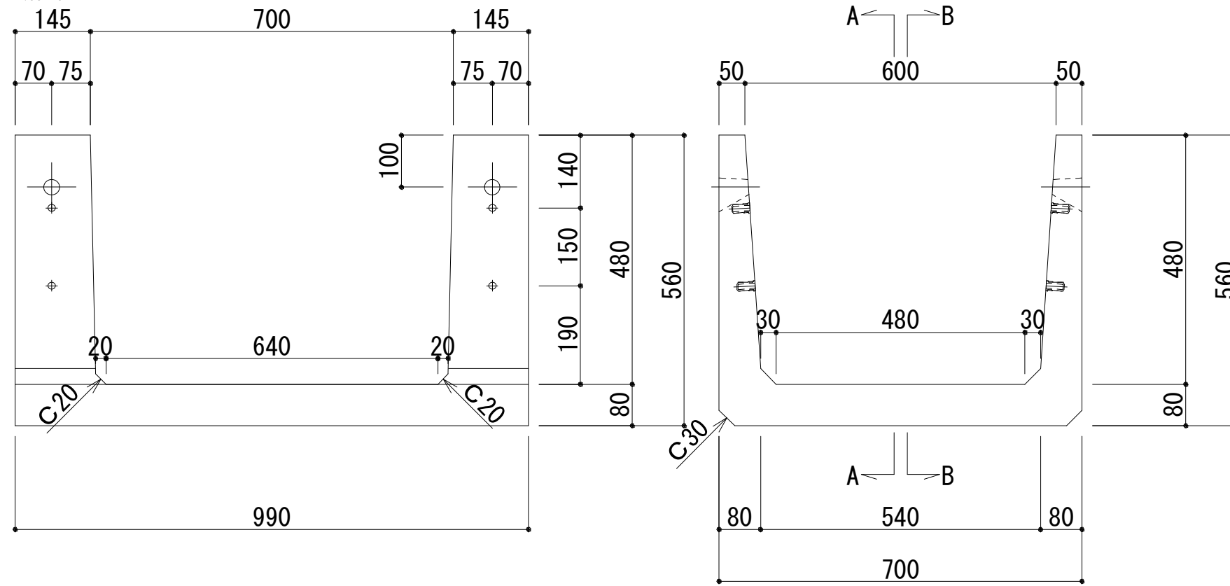
A-A 断面図
