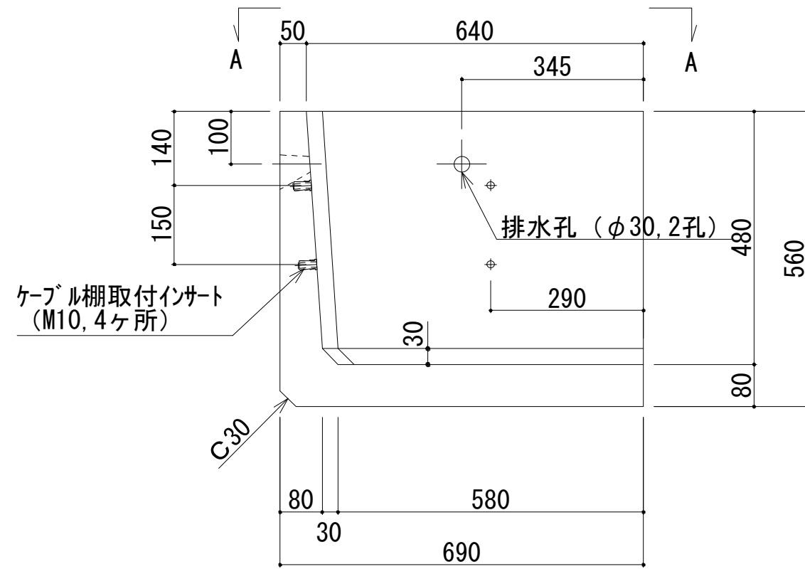
製品図
