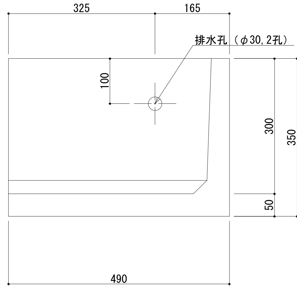
A-A 断面図
