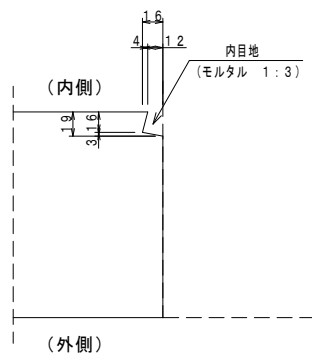
c部 (打設面) 内目地及びシーリング材貼付溝 拡大図 S=1:3
