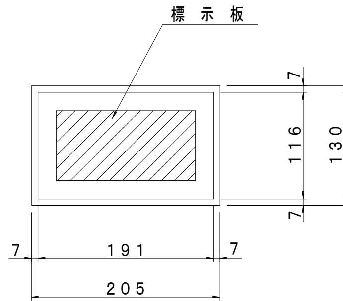
平面図
