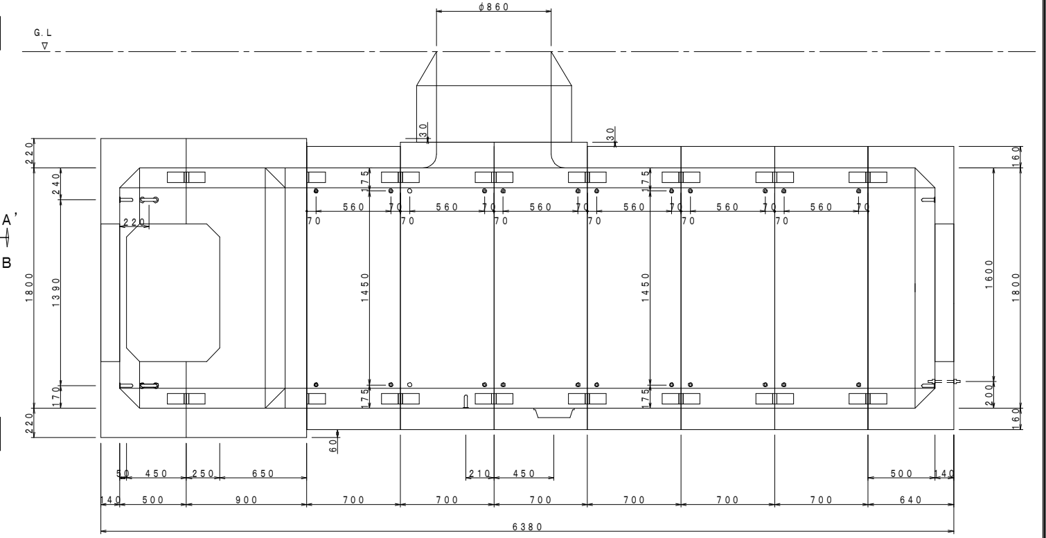
側面図 C-C'
