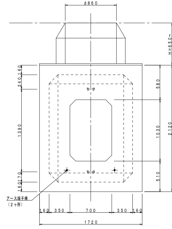
側面図 C-C'
