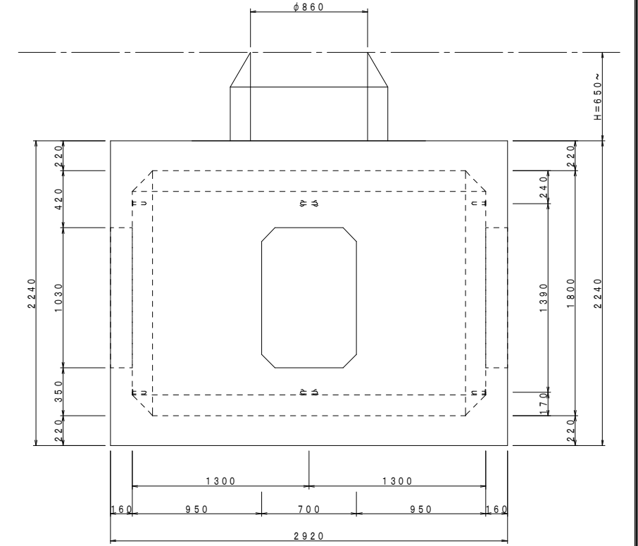
側面図 D-D'
