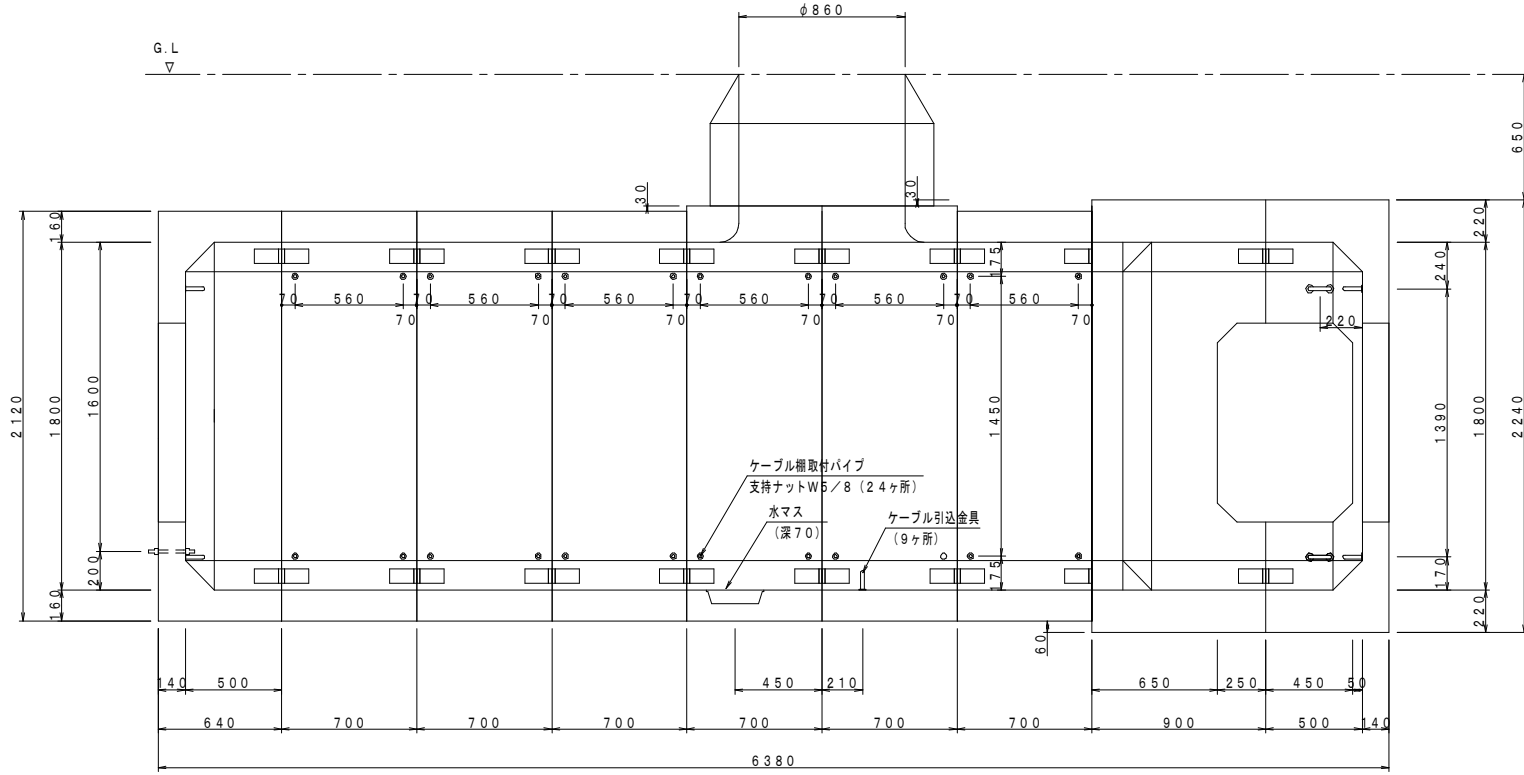
断面図 A-A'
