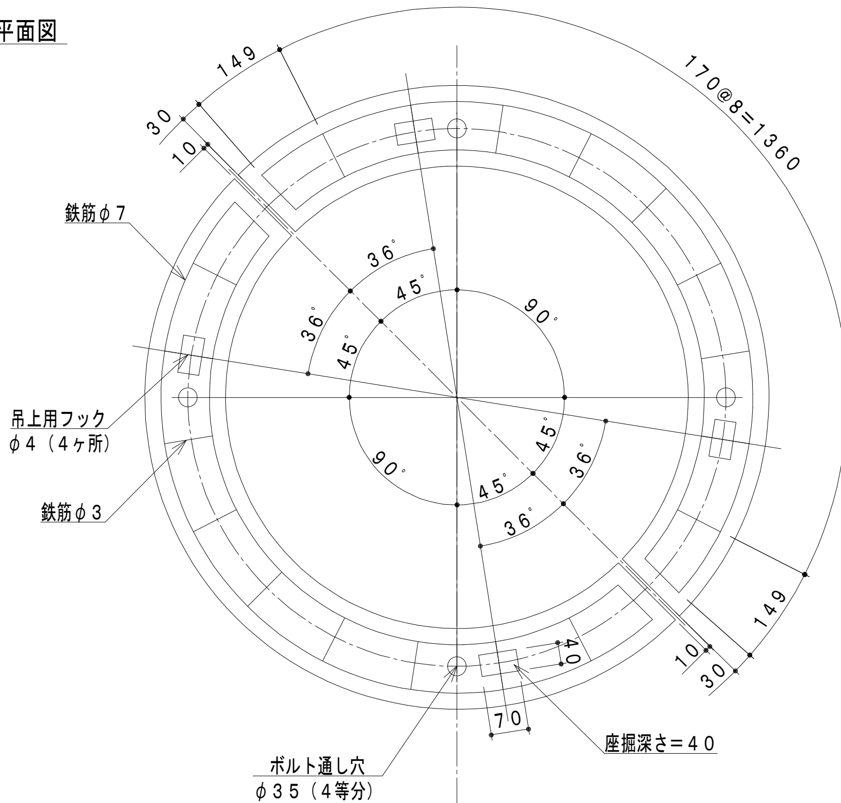
断面図
