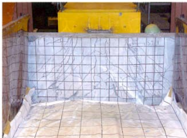
PCF壁高欄の破壊状況
