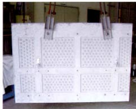
PCF版の外観（VFRCタイプ）
