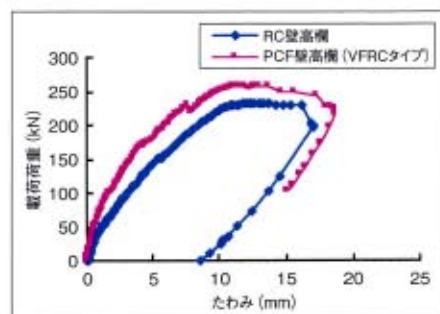
②PCF壁高欄 (VFRCタイプ)
