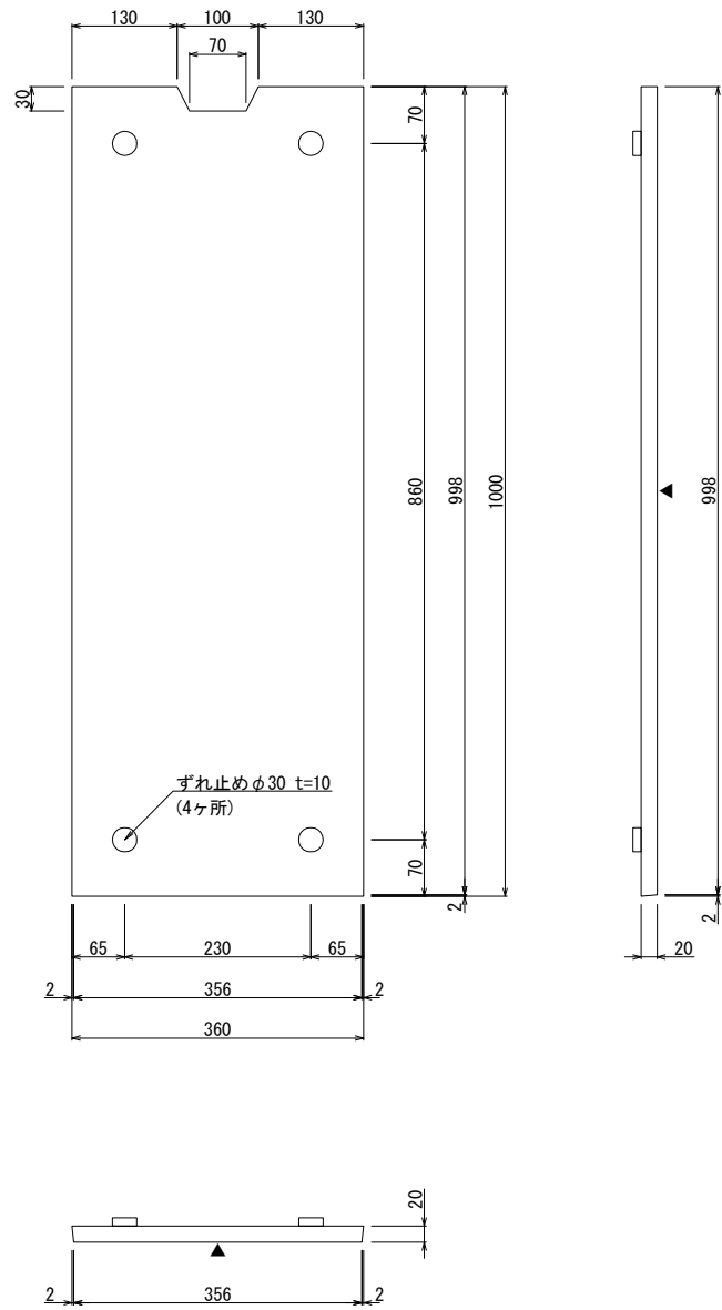
打設面視図
