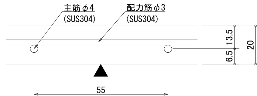
配筋断面詳細図
