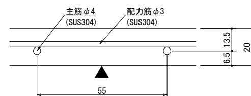
配筋断面詳細図
