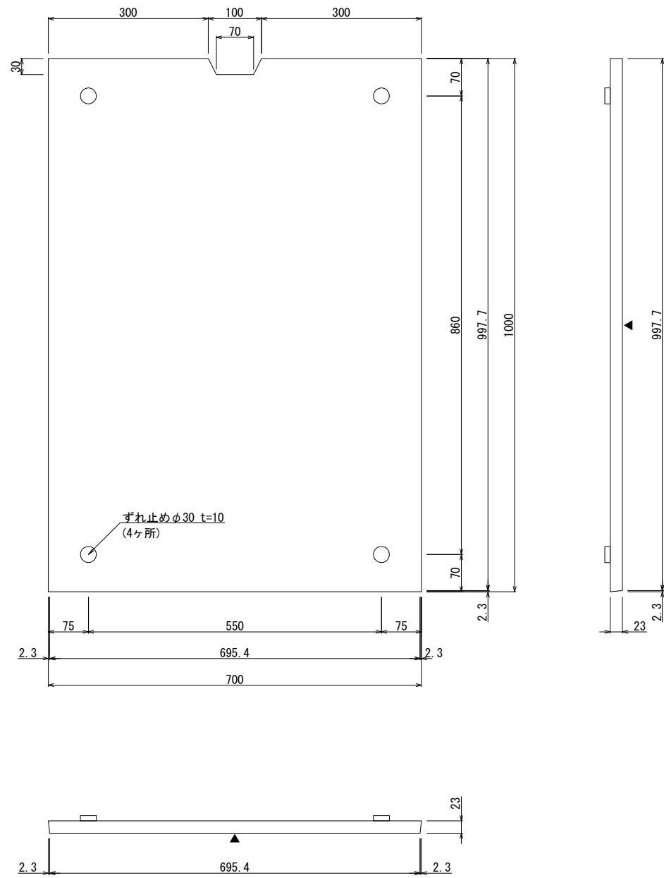
打設面視図
