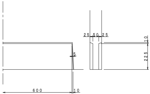
管路口詳細図
